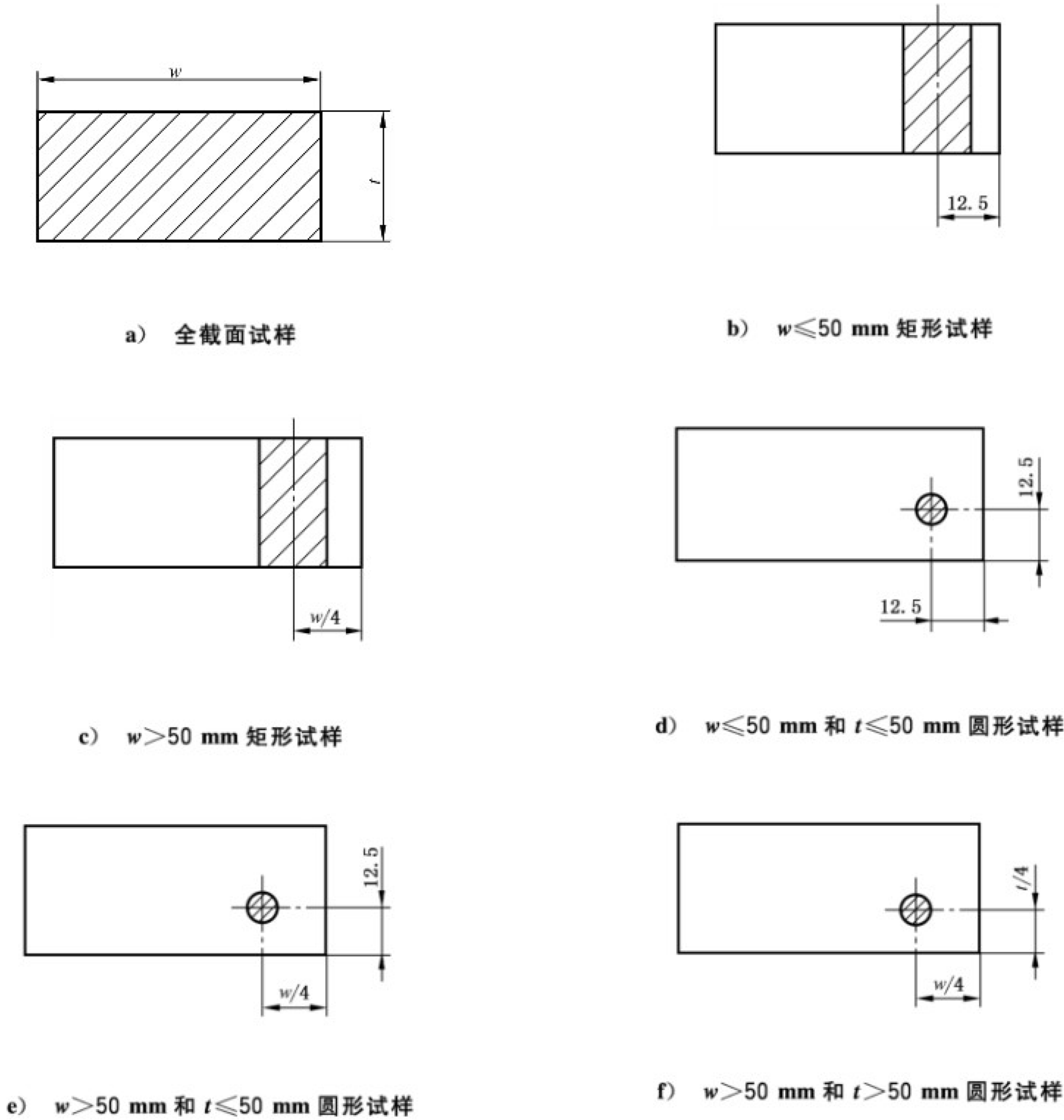
图 A.8 矩形截面条钢 拉伸试样的取样位置(见 A.5.1)
