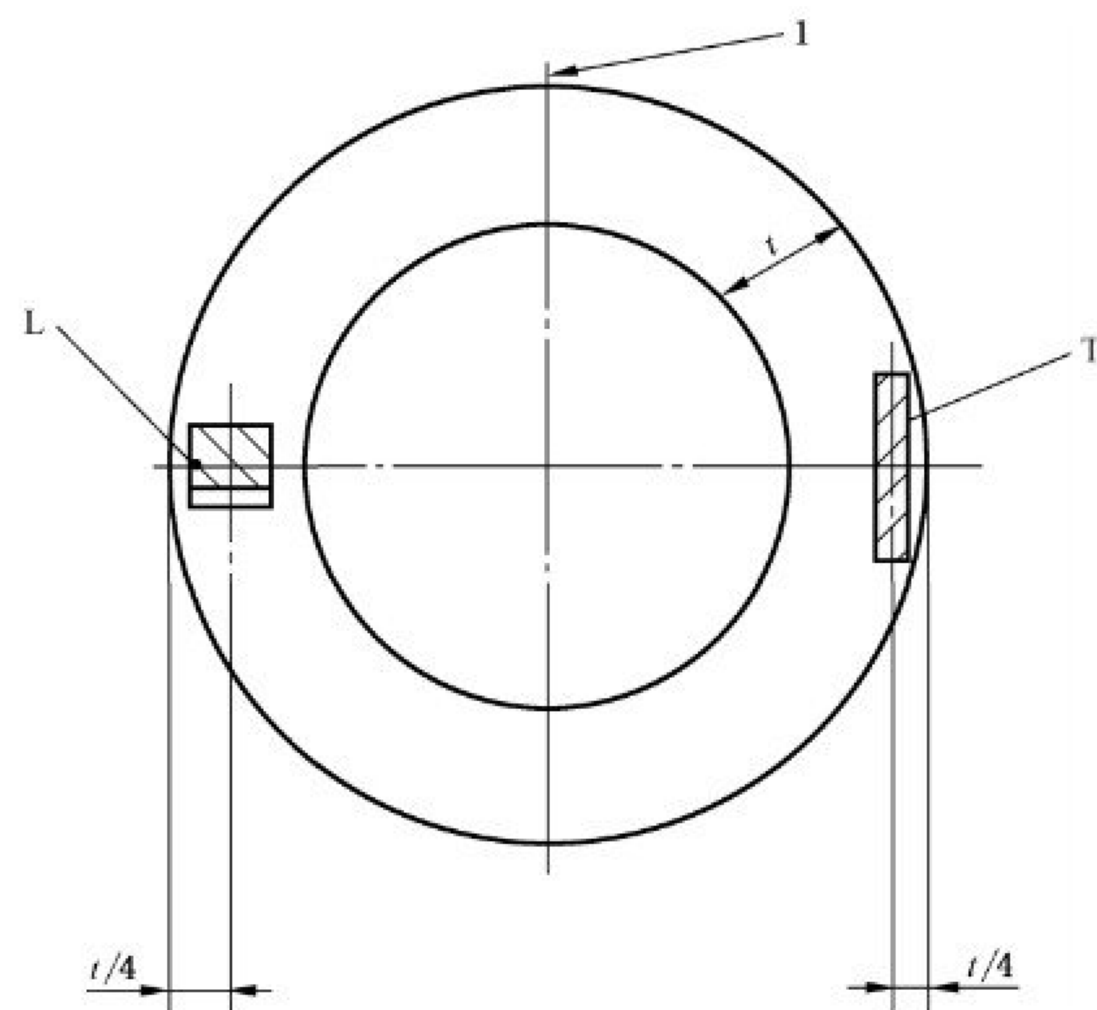
b) t > 40 mm 冲击试样
